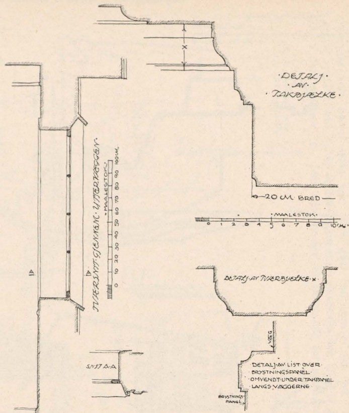
Detaljer fra Øier prestegaard. Efter opmaaling av arkitekt Herman Munthe-Kaas.
