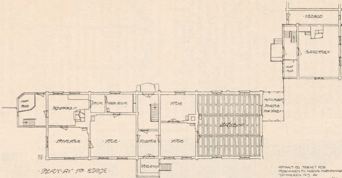
Øier prestegaard. Efter opmaaling av arkitekt Herman Munthe-Kaas
