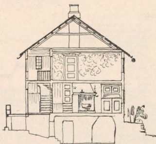
TVERRSNIT GÆNKENE BAARDSTUEN.
