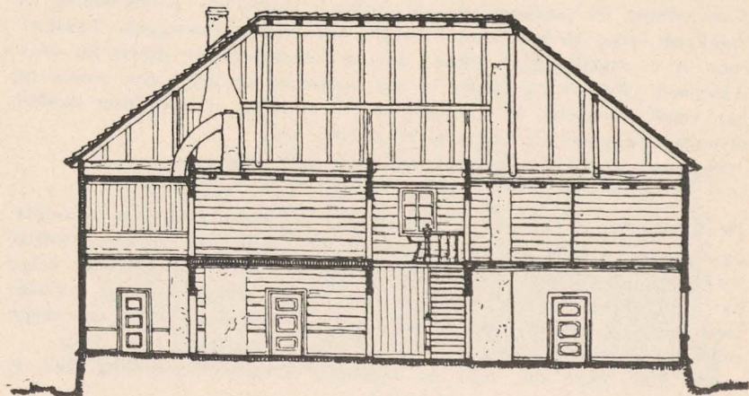
Snit B-B
