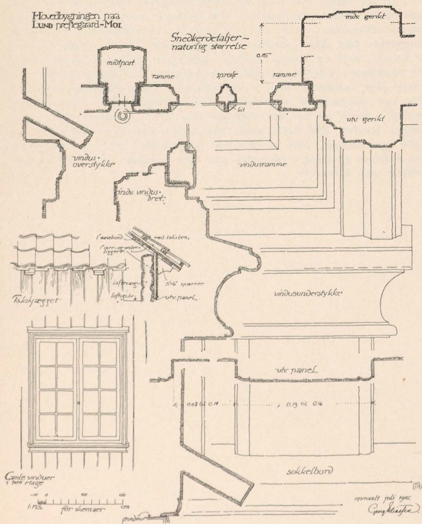
Detaljer av Lund prestegaard i Moi. Av arkitekt Georg Eliassen.
