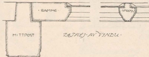
Detaljer fra Øier prestegaard. Efter opmaaling av arkitekt Herman Munthe-Kaas.
