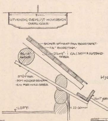
GESIMS I HOVEDBYGN.
